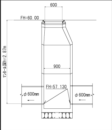
雨水マンホール構造図
